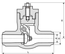
主要外形和链接尺寸 Main external and connectin dimensions
